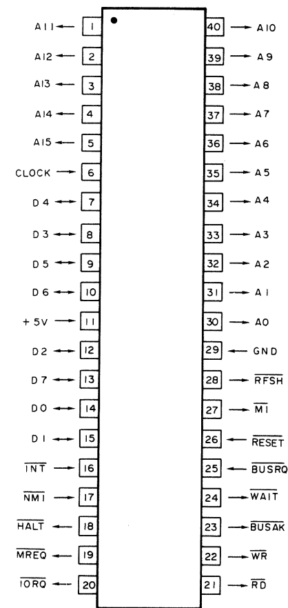
LH0080A
