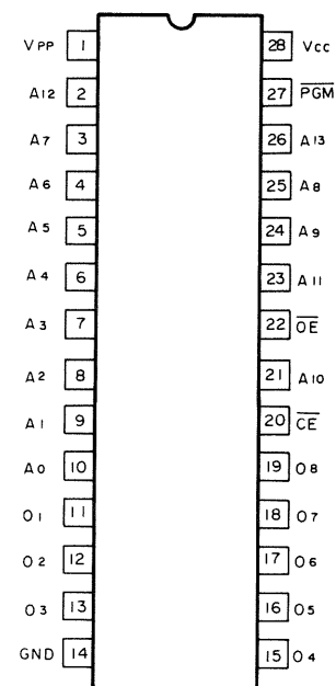
MBM27C128*S
