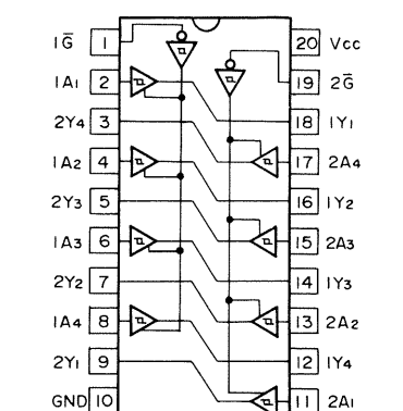
HD74LS244FP
