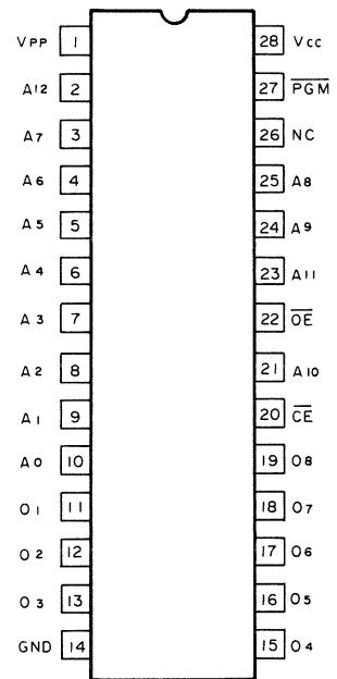
MBM27C64*U
