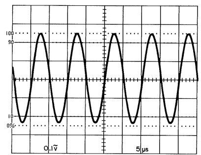
Fig. 24 DC - 5.0V Input 0.8Vp-p Sine Wave
