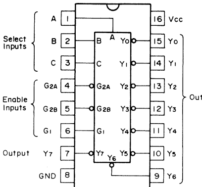
HD74LS138FP
