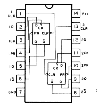
SN74ALS74AN
