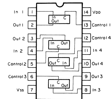
HD14066BFP
