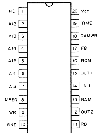
DTM-5010
