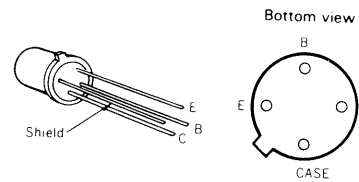
2SC1164 (O)*S
