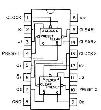
SN74ALS112AN
